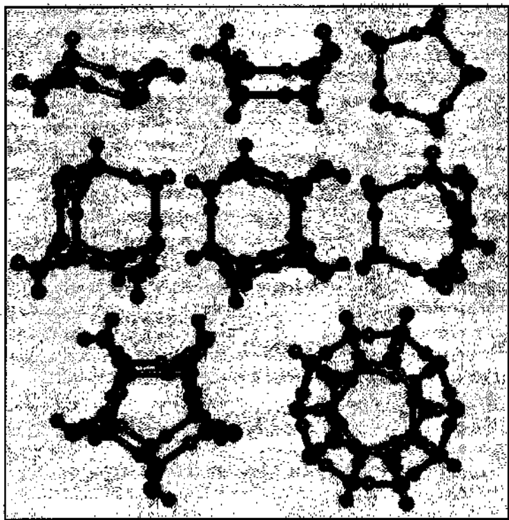
Рис. 3.2. Кластерная структура воды
