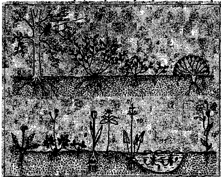
Рис. 4.15. Экологические группы растений по классификации К. Раункьера.
