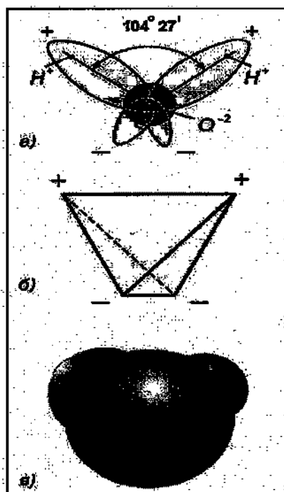
Рис. 3.1. Строение молекулы воды. а – положение атомов водорода и кислорода в молекуле воды; б и в – геометрические модели молекулы воды
