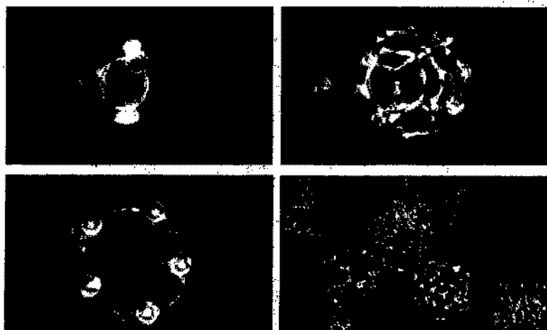
Рис. 3.4. Формирование сложных кластеров воды (компьютерное моделирование)
