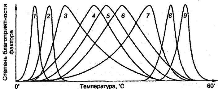
Рис. 2.2. Положение кривых оптимума на температурной шкале для разных видов.
